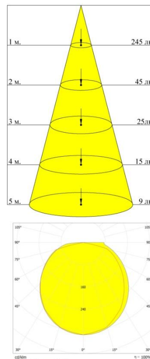
Рисунок 3 – Световое распределение.
