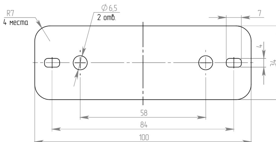
Рисунок 2 – Чертеж.
