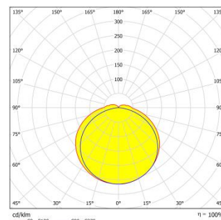
Рисунок 3 – Светораспределение светильника Geniled Лайнер-L 6W 5000К.
