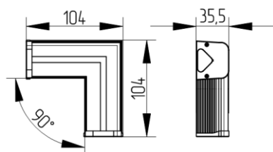
Рисунок 2 – Габаритные размеры светильника Geniled Лайнер-L 6W 5000К.
