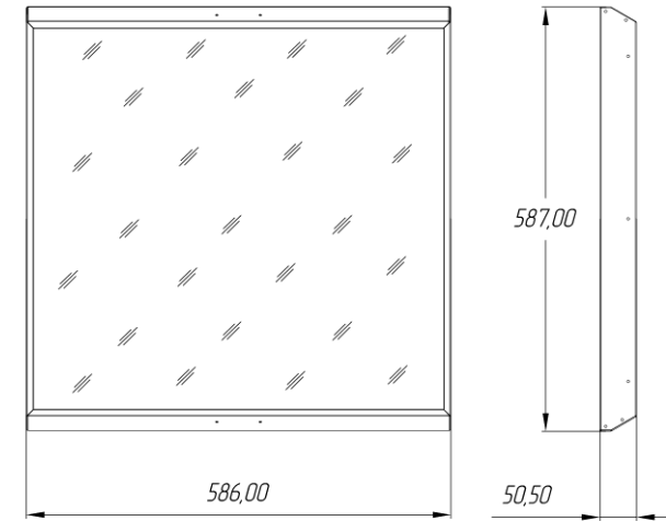
Рисунок 1. Габаритные размеры светильников серии ДПО10
