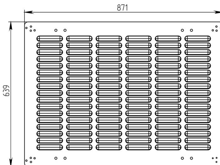
Рисунок 2 – Габаритный чертеж.
